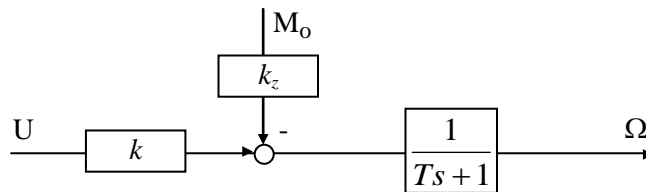
Model silnika sterowanego napięciowo
